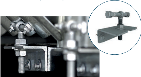
C1 Charnière pour capot rabattable
